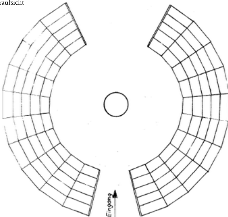
Aufbauplan: Draufsicht
