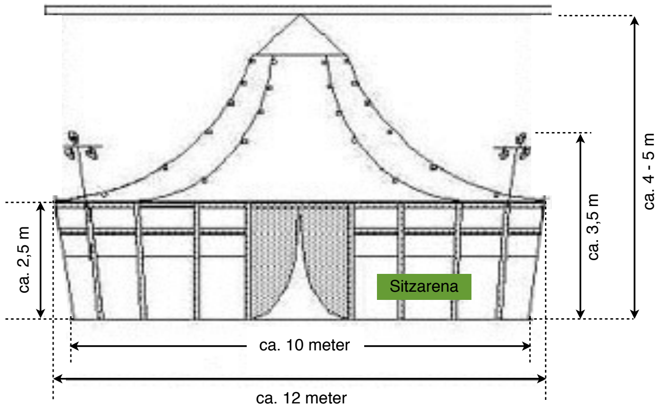
Aufbauplan: Seitenansicht
